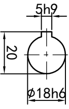
输出轴 細節A 比例2:1
