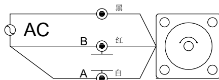
单相马达接线图
