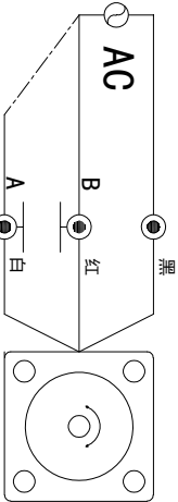
单相马达接线图
